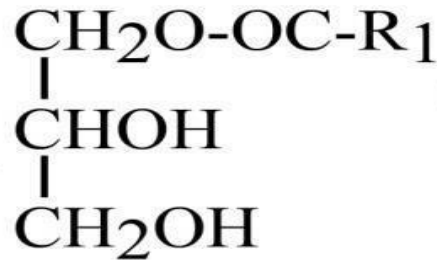
Monoglyceride
