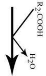
1,3-diglyceride
